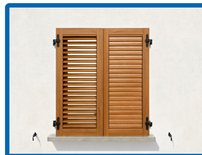
In battuta muro, cerniera a croce regolabile
